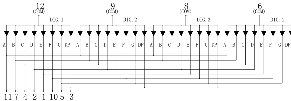
KW4-S391AVA
